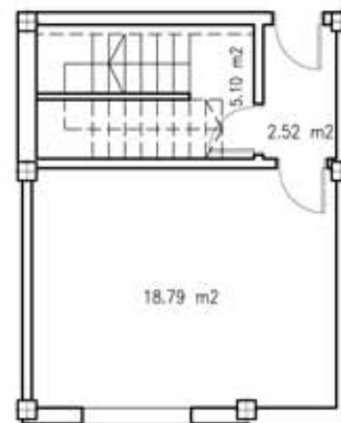
SOTANO COMUNICADO
