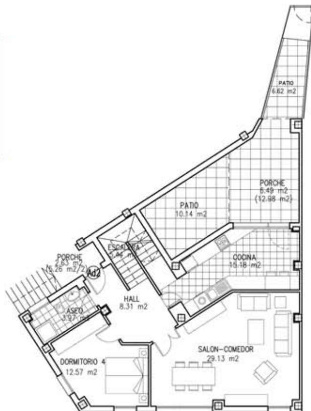
PLANTA BAJA
