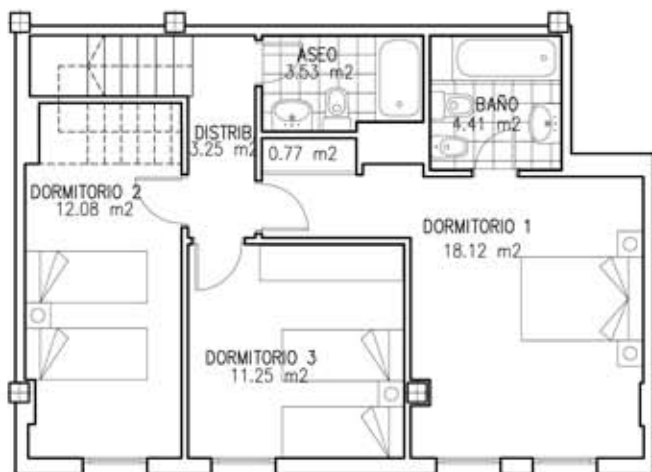
PLANTA PRIMERA
